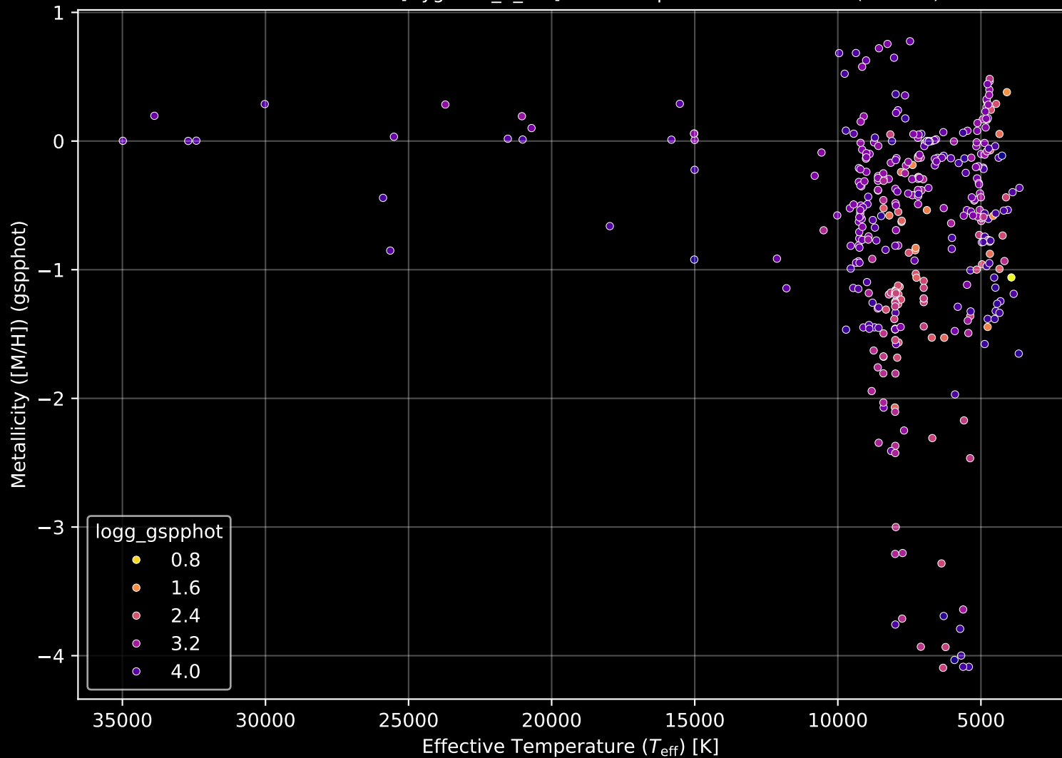
APOGEE DR17 Field: [CygnusX_S_btx] Stellar Population Parameters (n= 372)
